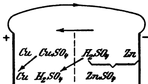
Abb. 68. Daniellsche Zelle.
